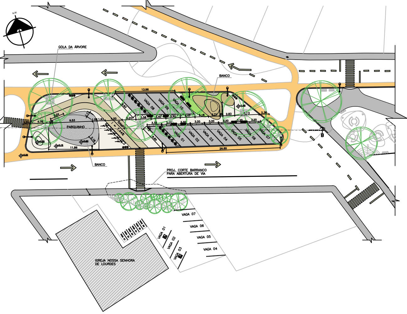
PLANTA TÉCNICA PRAÇA ESTACIONAMENTO ESCALA 1:200
