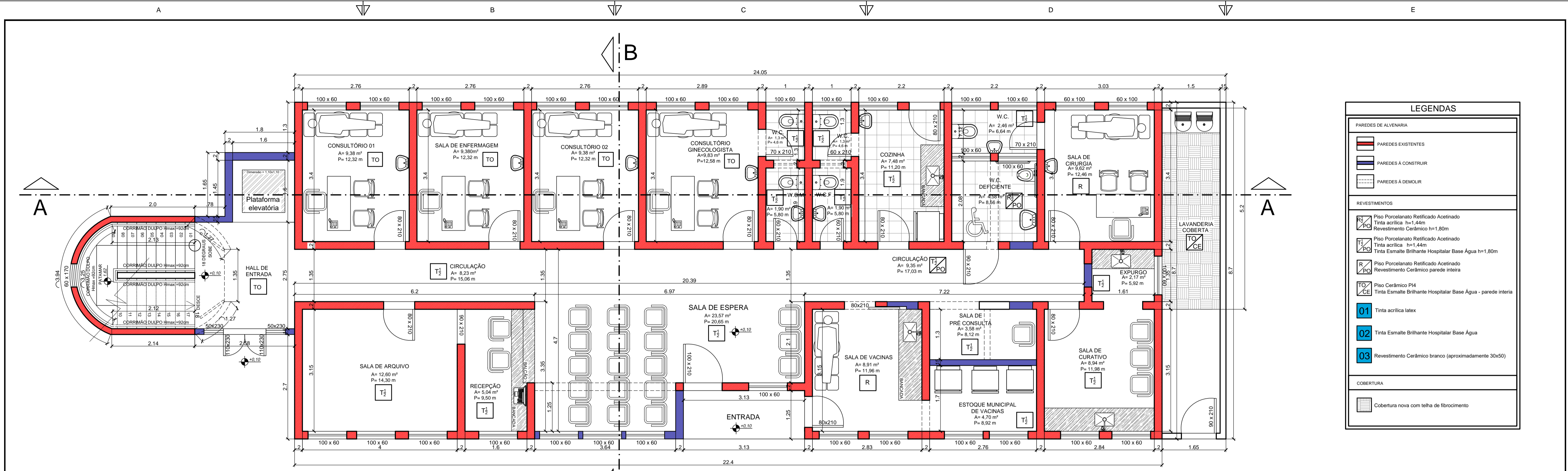
PLANTA BAIXA PAVIMENTO TÉRREO ESC. 1/50 ÁREA: 214,67 m 2
